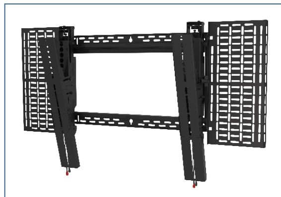
(2) Support de composant universel ACC-UCM illustré avec le support universel SmartMount® à croisillon et montage mural (STS650)
