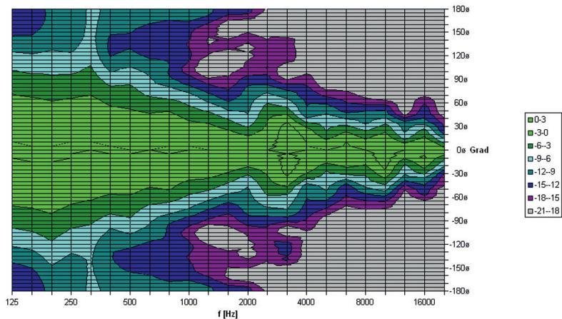
RL 204 SN vert. Direktivität Plot
