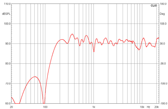
ZL 100 hor. Direktivität Plot
